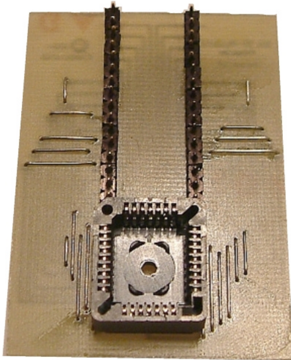
Bestückungsseite
