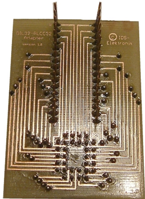
Lötseite
